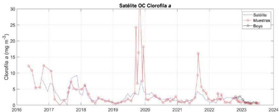
Figura 14: Comparación de las series temporales de clorofila a de los datos satelitales, muestreos DMMEM y boya SMLG.
