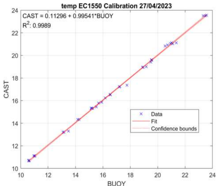
Figura 21: Calibración de la temperatura del sensor de conductividad (EC-1550) de la boya SMLG - 14/10/2023 a 07/05/2023.
