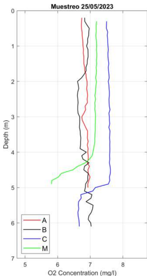
Figura 47: Perfiles de Concentración de Oxígeno obtenidos el día 25/05/2023 con el CTD.
