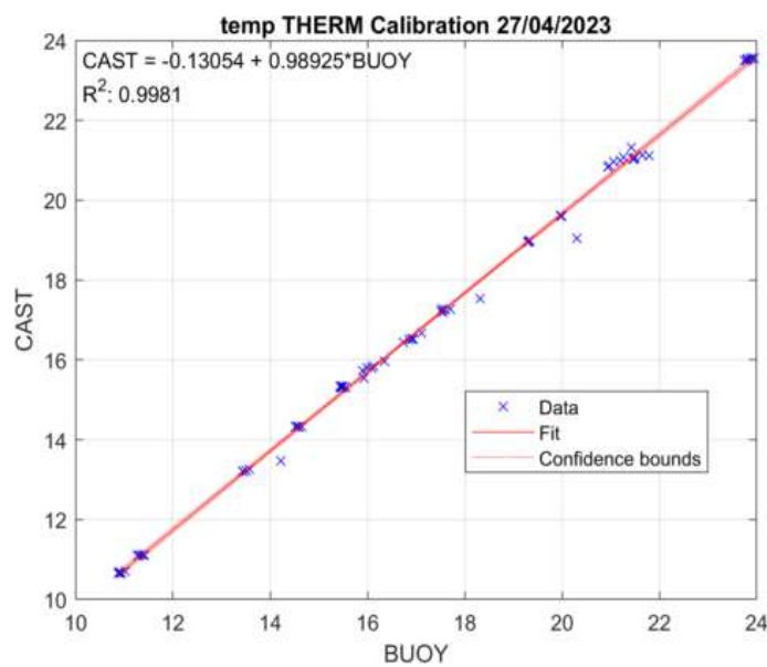
Figura 17: Calibración de los datos de temperatura de los Termistores de la boya SMLG - 14/10/2023 a 07/05/2023.
