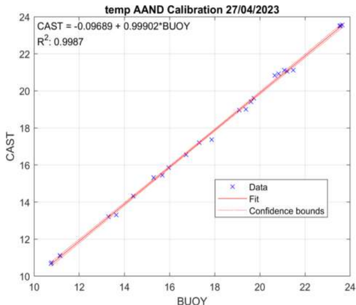
Figura 19: Calibración de los datos de temperatura de los sensores de oxígeno Aanderaa de la boya SMLG - 14/10/2023 a 07/05/2023.
